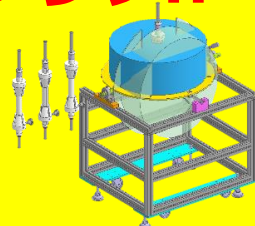
前段取り替え治具・シャフト3本
